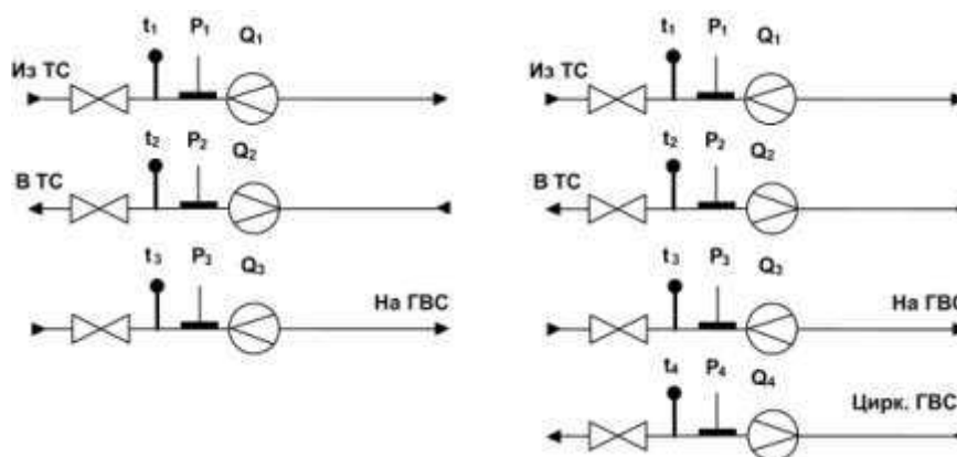
Рис.4. Схемы теплотребления с подпиткой из различных трубопроводов
